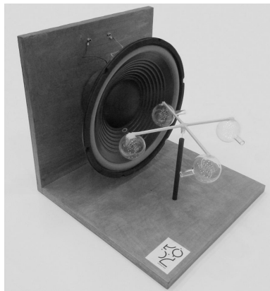
Fot. 1. Karuzela Helmholtza. „Ramię” przyrządu wykonano z dwóch kawałków sklejk – poziomego i pionowego – głośnik przyklejono bezpośrednio do pionowego kawałka. Łożysko wirnika stanowi mała próbówka, odwrócona dnem do góry i przyklejona od dołu do krzyżaka. Wirnik opiera się na ostrzu igły, wprowadzonej do próbówki i osadzonej tym końcem we wsporniku, który osadzono w poziomym kawałku sklejk.
