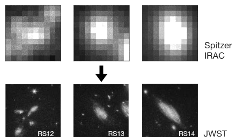
Porównanie zdjęć trzech czerwonych galaktyk spiralnych pochodzących z teleskopu kosmicznego Spitzera i nowego teleskopu kosmicznego Jamesa Webba
